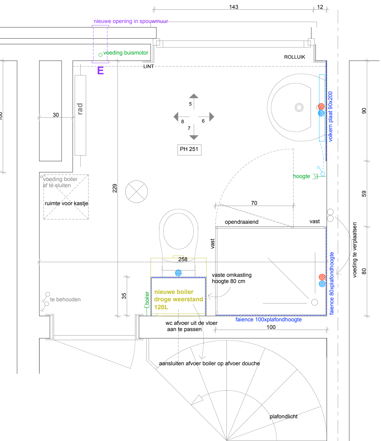
GRONDPLAN BADKAMER
