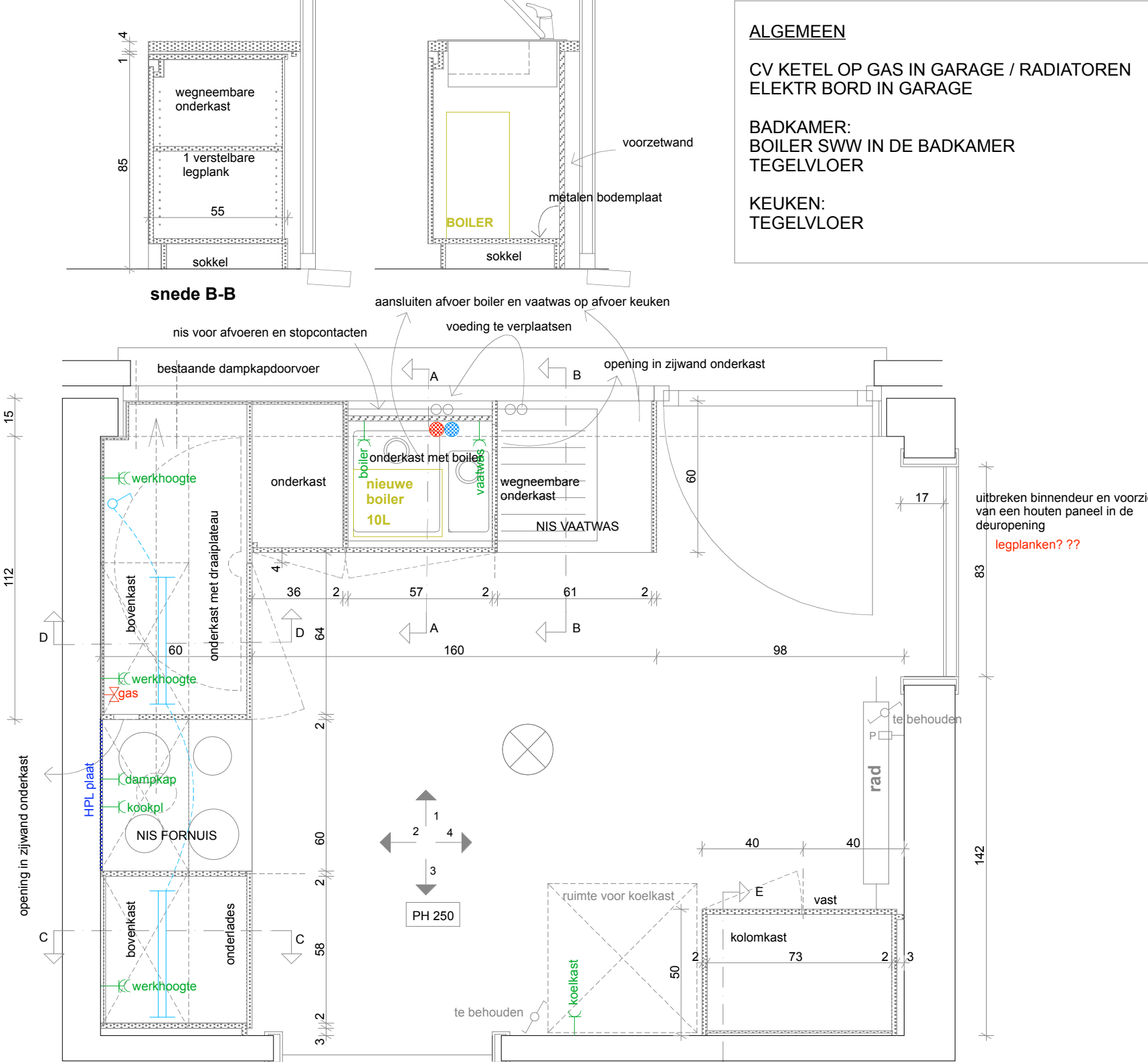
GRONDPLAN KEUKEN
