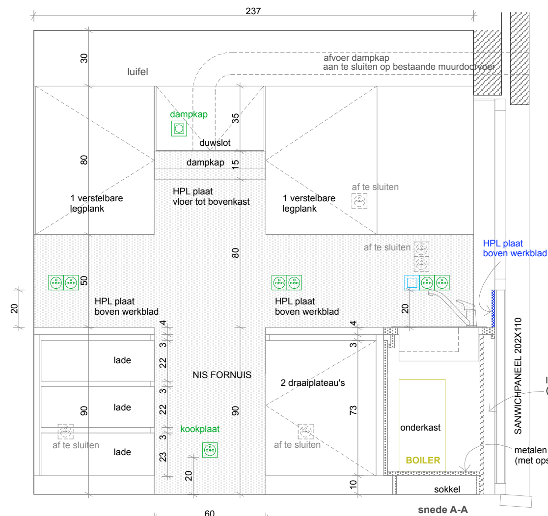
AANZICHT 2 snede A-A
