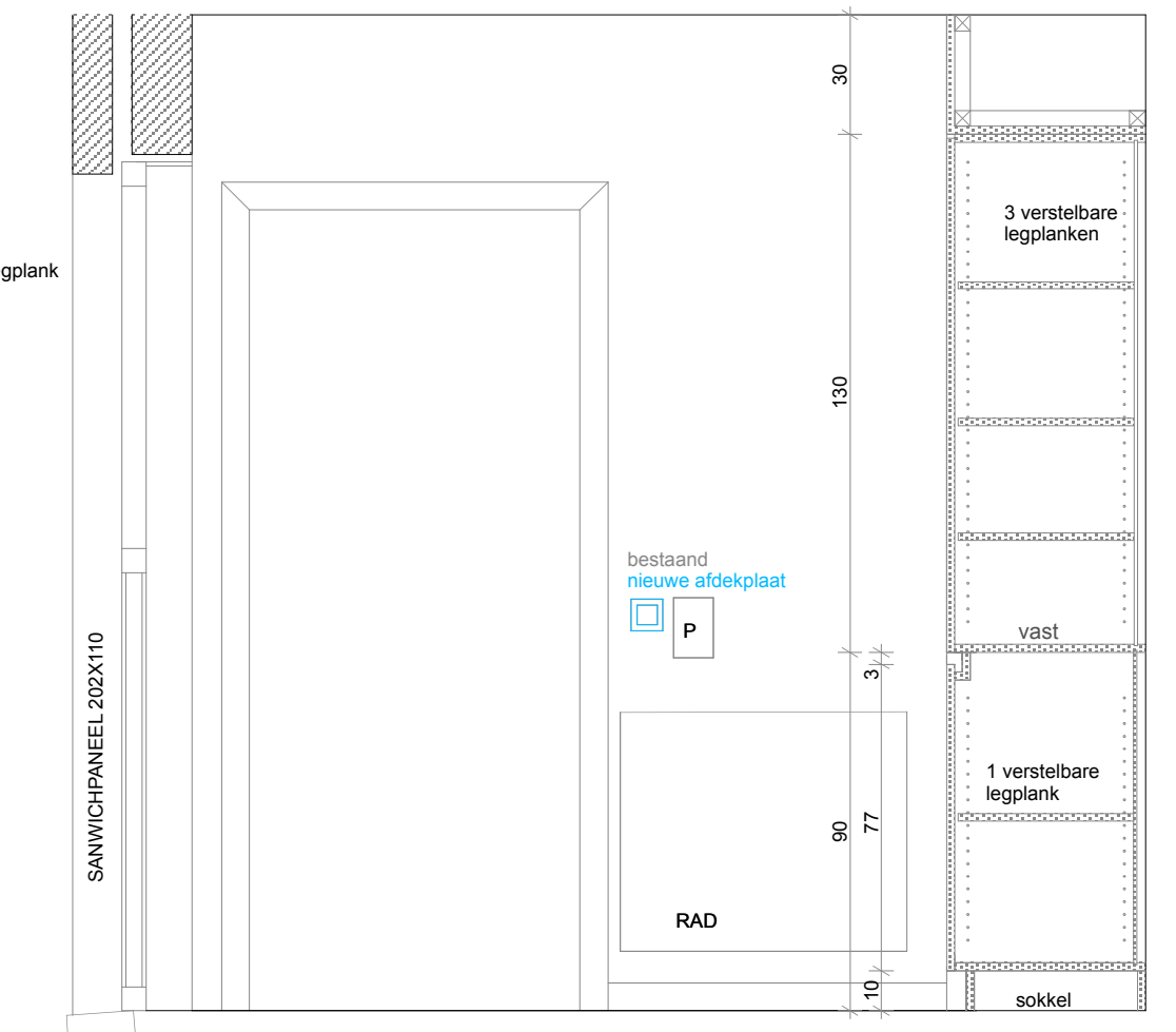
AANZICHT 4 snede E-E
