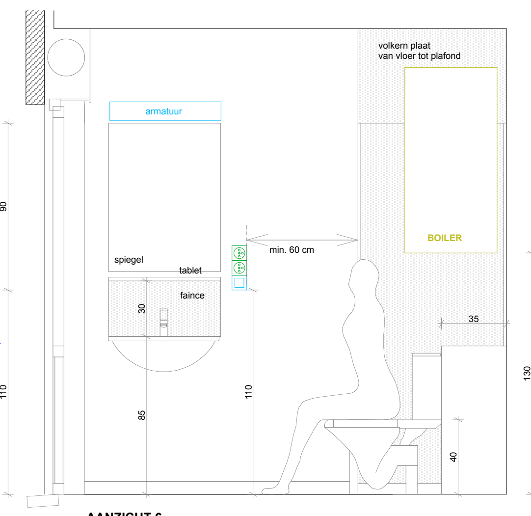
AANZICHT 6
