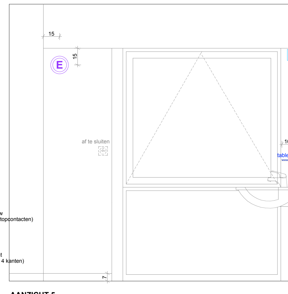
AANZICHT 5
