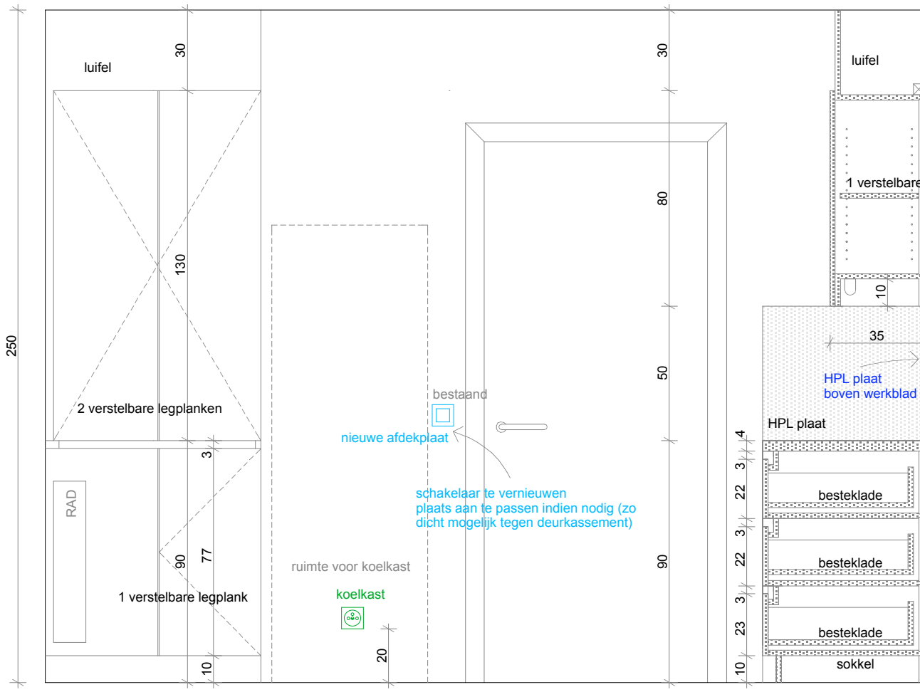
AANZICHT 3 snede C-C
