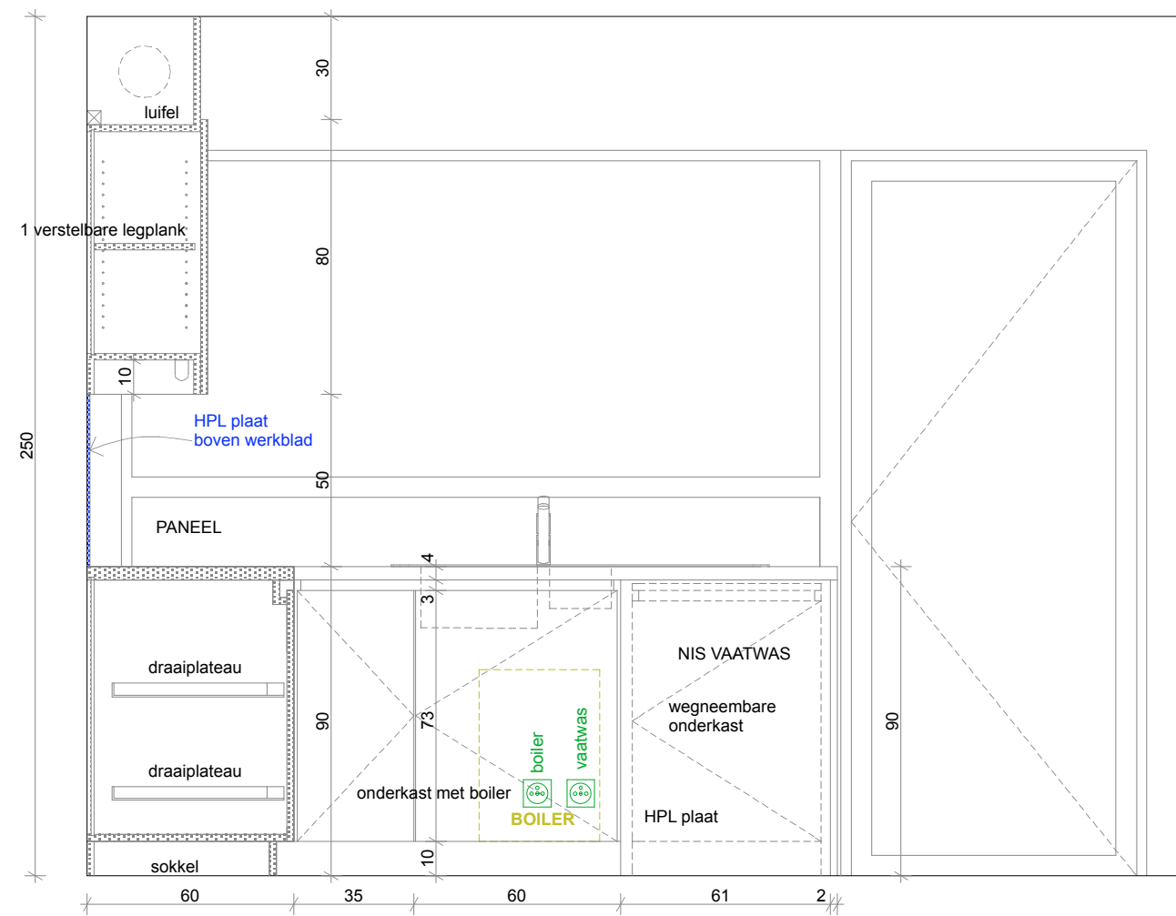
snede D-D AANZICHT 1
