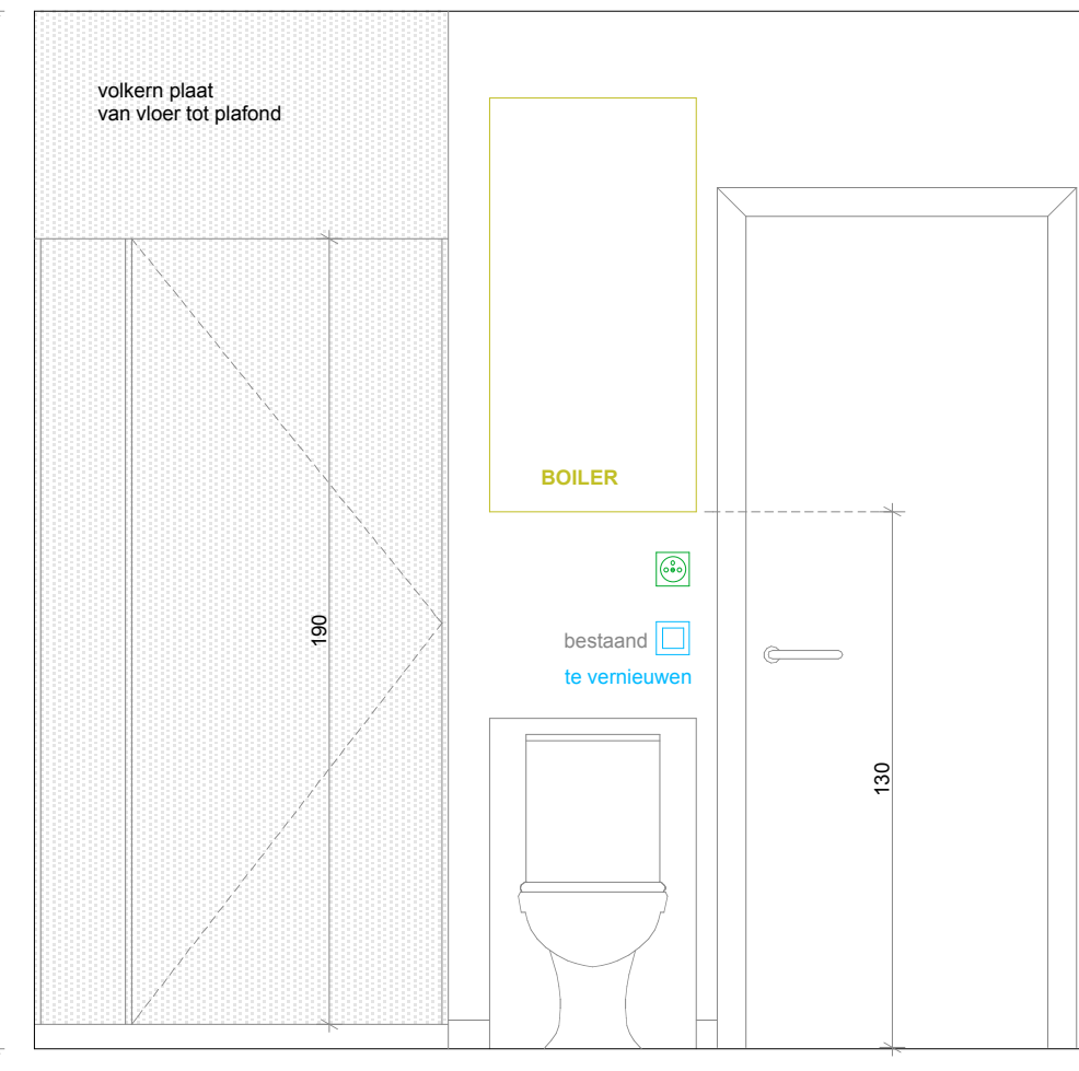
AANZICHT 7
